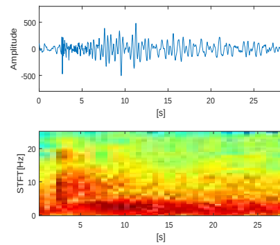
(d) Hybrid Event (HYB)
