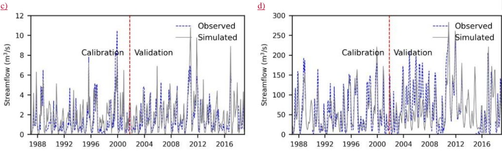
Figure 3 Monthly calibration and validation for streamflow at: a) Puente Salguero, b) Puente Carretera, c) Cantaclaro and d) Puente Canoas.
