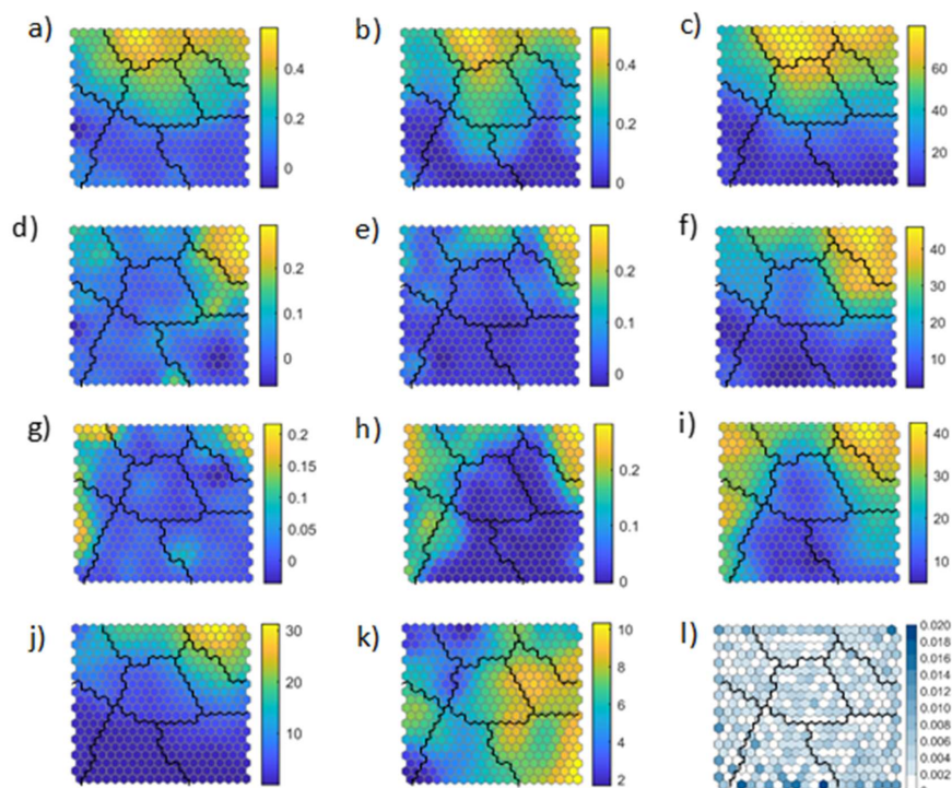
Figure 9: SOM classification: a) \tau_1(Q-P) , b) \tau_2(P-Q) , c) JO(Q-P) , d) \tau_1(Q-SW) , e) \tau_2(SW-Q) , f) JO(Q-SW) , g) \tau_1(P-SW) , h) \tau_2(SW-P) , i) JO(P-SW) , j) JQ(Q-P-SW) , k) SI , l) probability of each SOM centroid.
