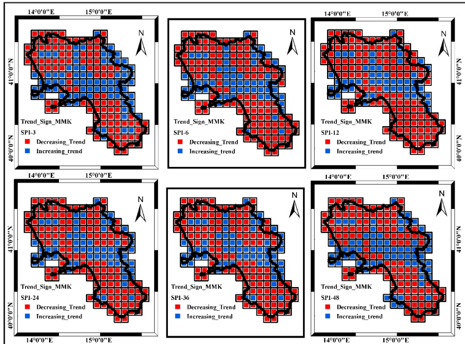
230 Figure 4: SPI MMK test sign, for the different accumulation scales ( \alpha = 5\% ). Trasforma le frecce in colori (se vuoi anche come la figura seguente) perché continua ad essere difficile la visione distinta.
