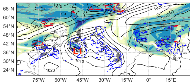
(d) 07 Jan 2021 12 UTC
