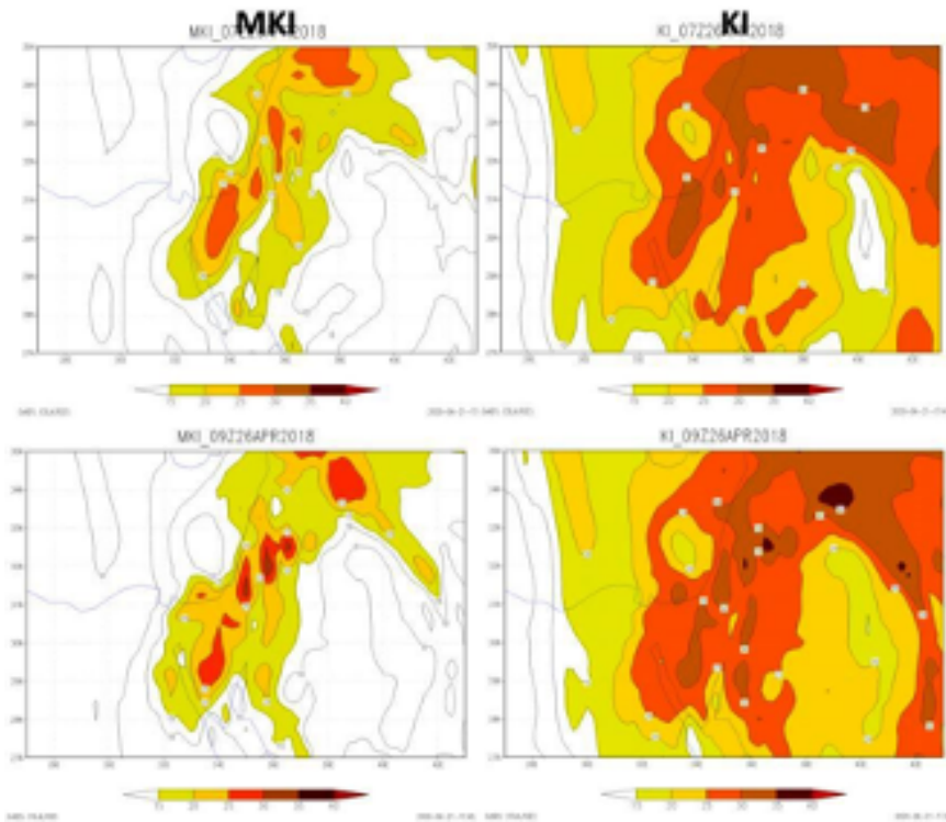
Fig. 3. MKI vs. KI
