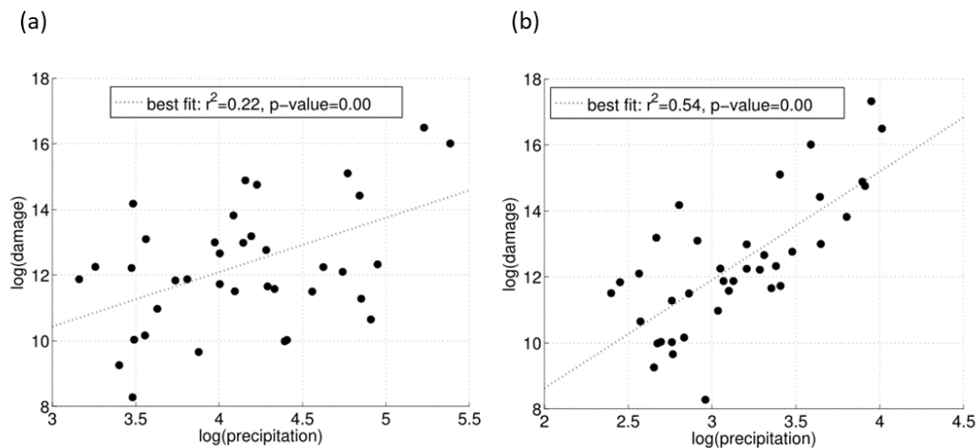
Fig. 6. Scatter plot (a) damages (D) versus 24 h precipitation and (b) damages (D) versus 30 minute precipitation.
