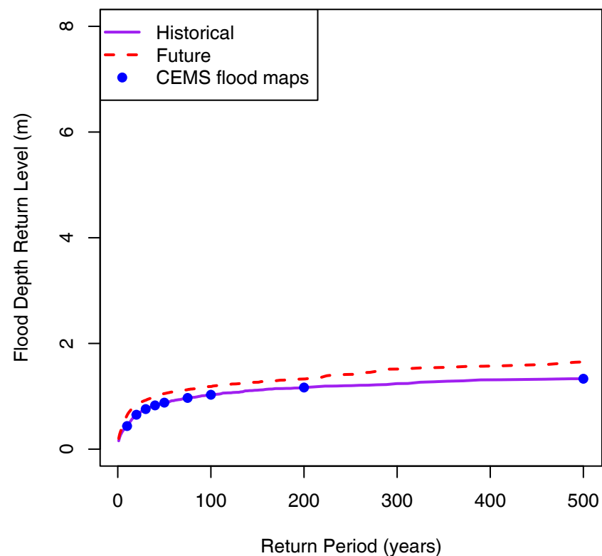
(d) Edinburgh: Flood depth return level curve
