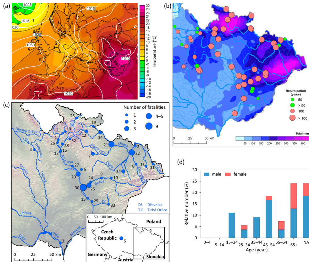
Figure 8. The flood of July 1997 in the eastern part of the Czech Republic: (a) sea level pressure (hPa) and air temperature at the 850 hPa level on 6 July at 18:00 UTC (Wetterzentrale, 2026); (b) precipitation totals on 5–8 July 1997 and N -year return period of peak discharges Q_N \geq 50 years for hydrological stations of the CHMI (Brázdil et al., 2019); (c) municipalities with fatalities (number in brackets): 1 – Bohdík (1), 2 – Bohumín (1), 3 – Břeclav (1), 4 – Česká Třebová (1), 5 – Český Šternberk (2), 6 – Dolany (1), 7 – Dvorce (2), 8 – Frýdek-Místek (1), 9 – Hranice (1), 10 – Hustopeče nad Bečvou (1), 11 – Jindřichov (1), 12 – Karlovice (2), 13 – Komorní Lhotka (1), 14 – Krnov (2), 15 – Kroměříž (1), 16 – Lesnice (1), 17 – Leština (1), 18 – Město Albrechtice (1), 19 – Nové Losiny (1), 20 – Olomouc (3), 21 – Opava (4), 22 – Ostrava (5), 23 – Písečná (1), 24 – Prosenice (1), 25 – Přerov (3), 26 – Ruda nad Moravou (1), 27 – Střeň (1), 28 – Šumperk (1), 29 – Tlumačov (1), 30 – Troubky (9), 31 – Třinec (1), 32 – Vernířovice (1), 33 – Zádveřice-Raková (1), 34 – Závěšice (2); (d) distribution of fatalities according to sex and age.
