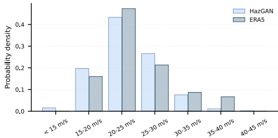
(d) Gumbel
