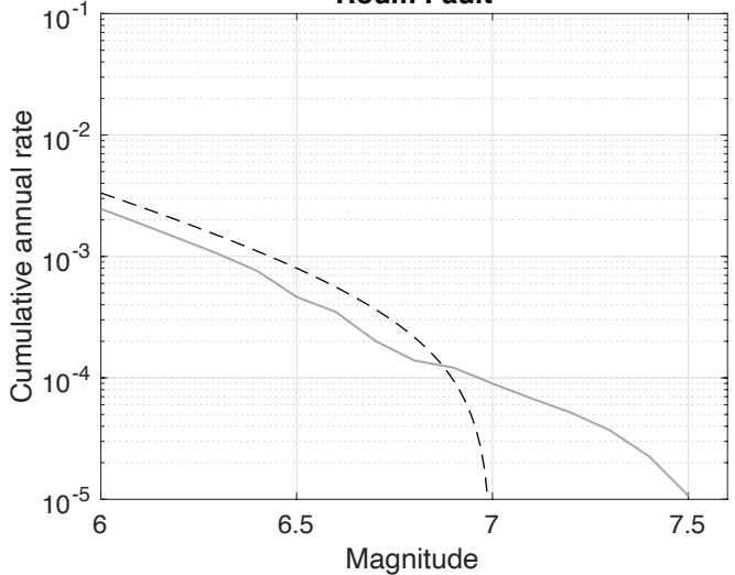
Roum Fault
