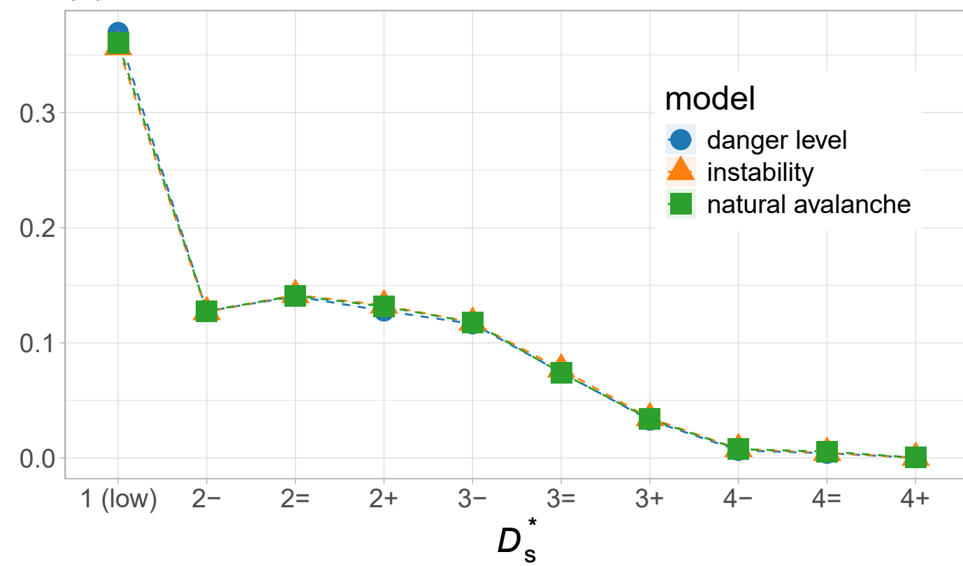
(d) Events (natural avalanches)
