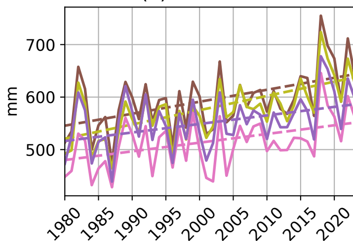
(d) Potential ET
