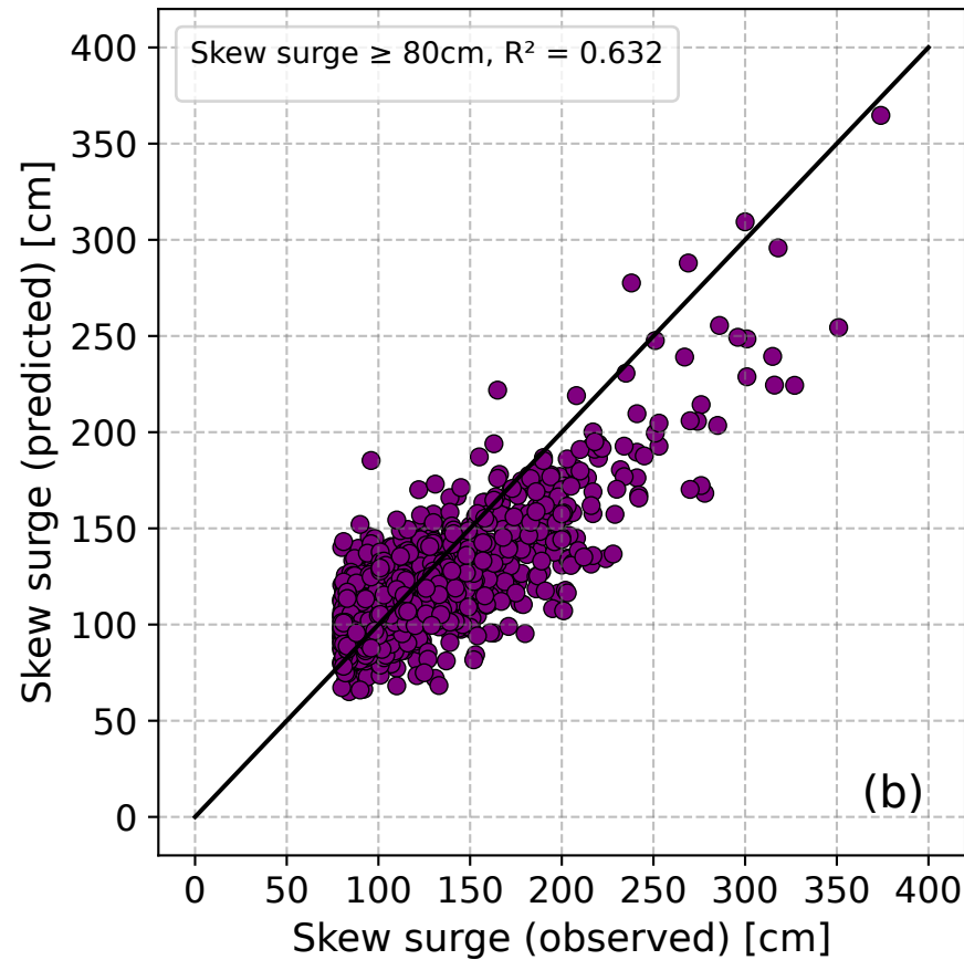
Lasso regression
