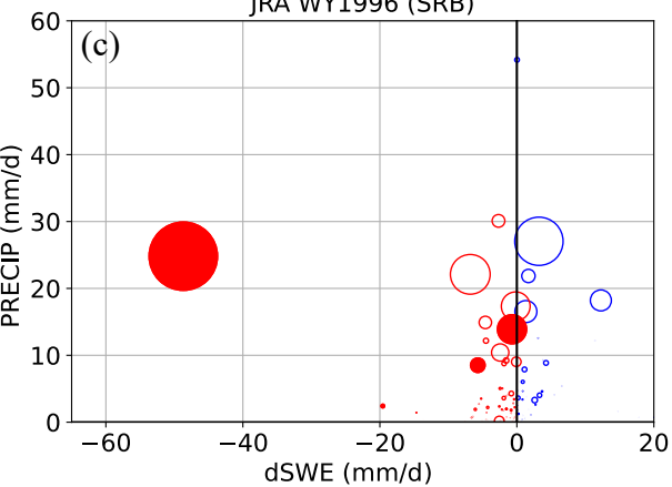
JRA WY1996 (SRB)
