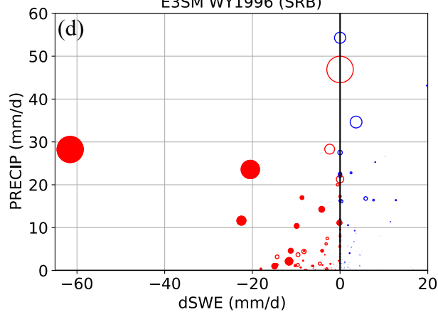
E3SM WY1996 (SRB)
