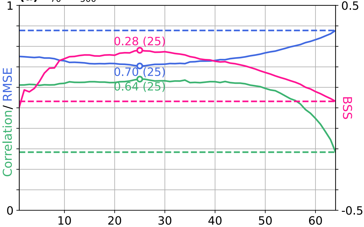
(b) T_{70}
