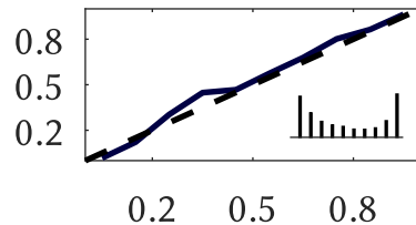
GoogLeNet
