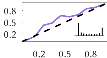
Logreg
