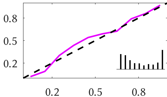
LASSO
