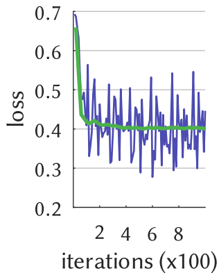
GoogLeNet
