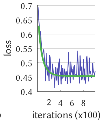
Logreg
