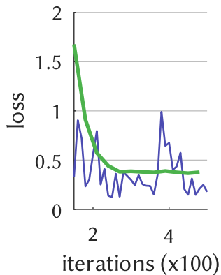
GoogLeNet
