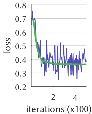
Logreg
