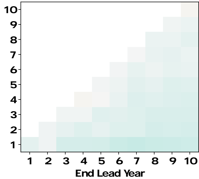
(d) Low Storm Activity
