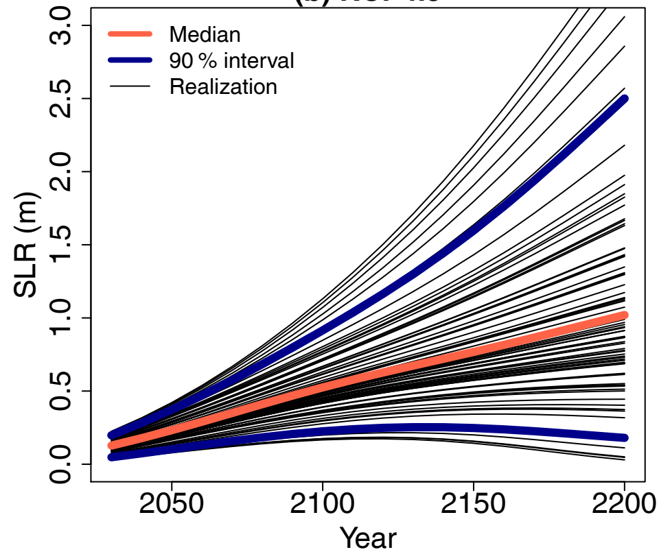
(b) RCP4.5
