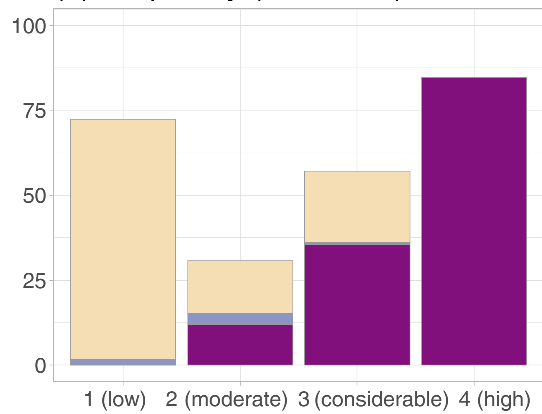
(d) frequency (wet snow)
