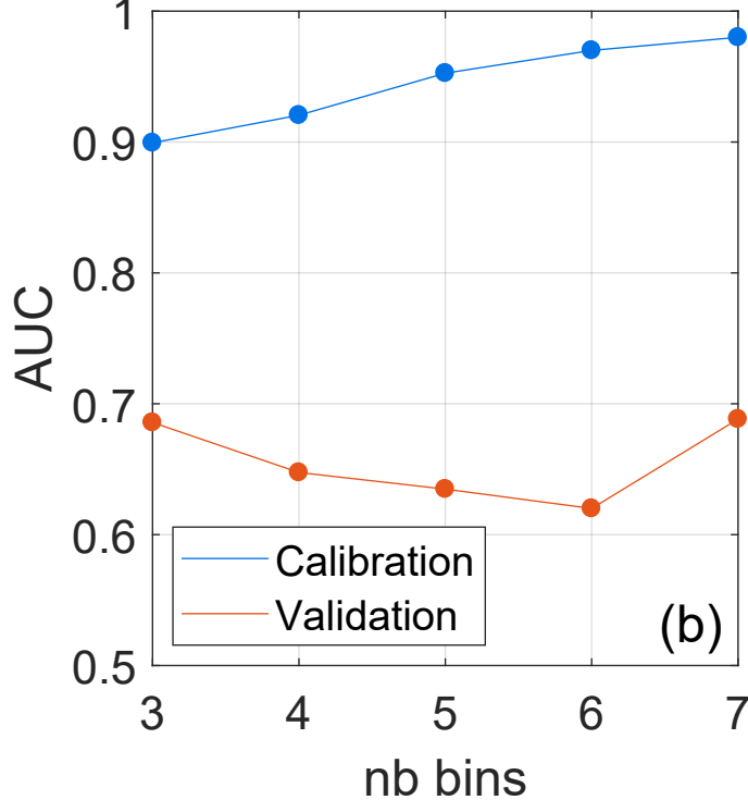
AUC
