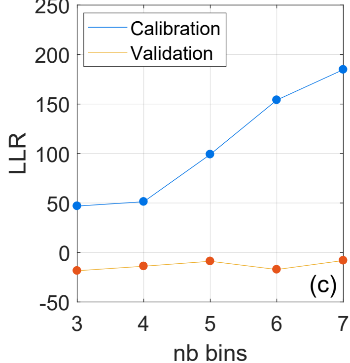
\Sigma LLR
