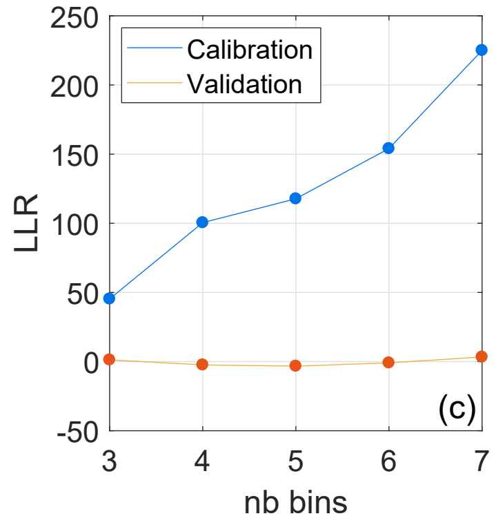
\Sigma LLR
