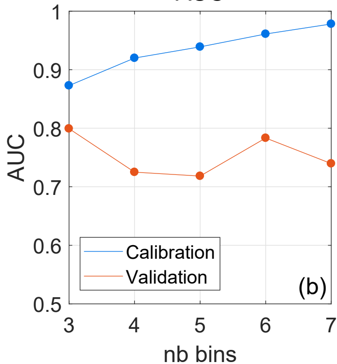
AUC
