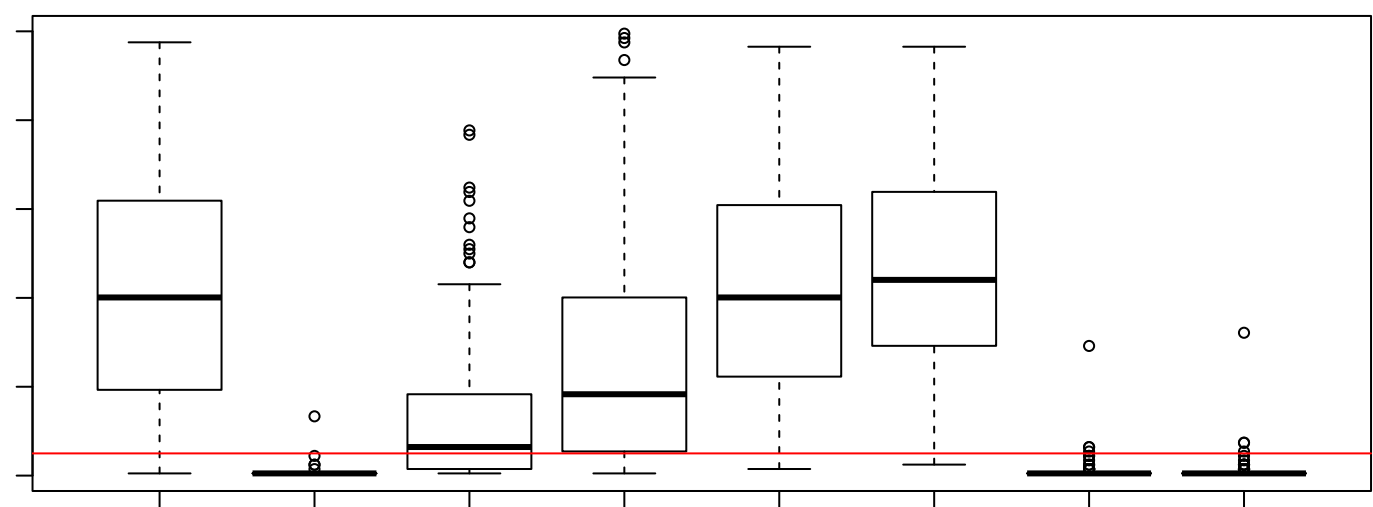
(d) Precipitation deficit and discharge deficit
